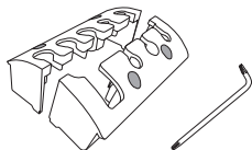
Komora przewodu (2 sztuki) i wbudowane śruby wraz ze śrubokrętem
