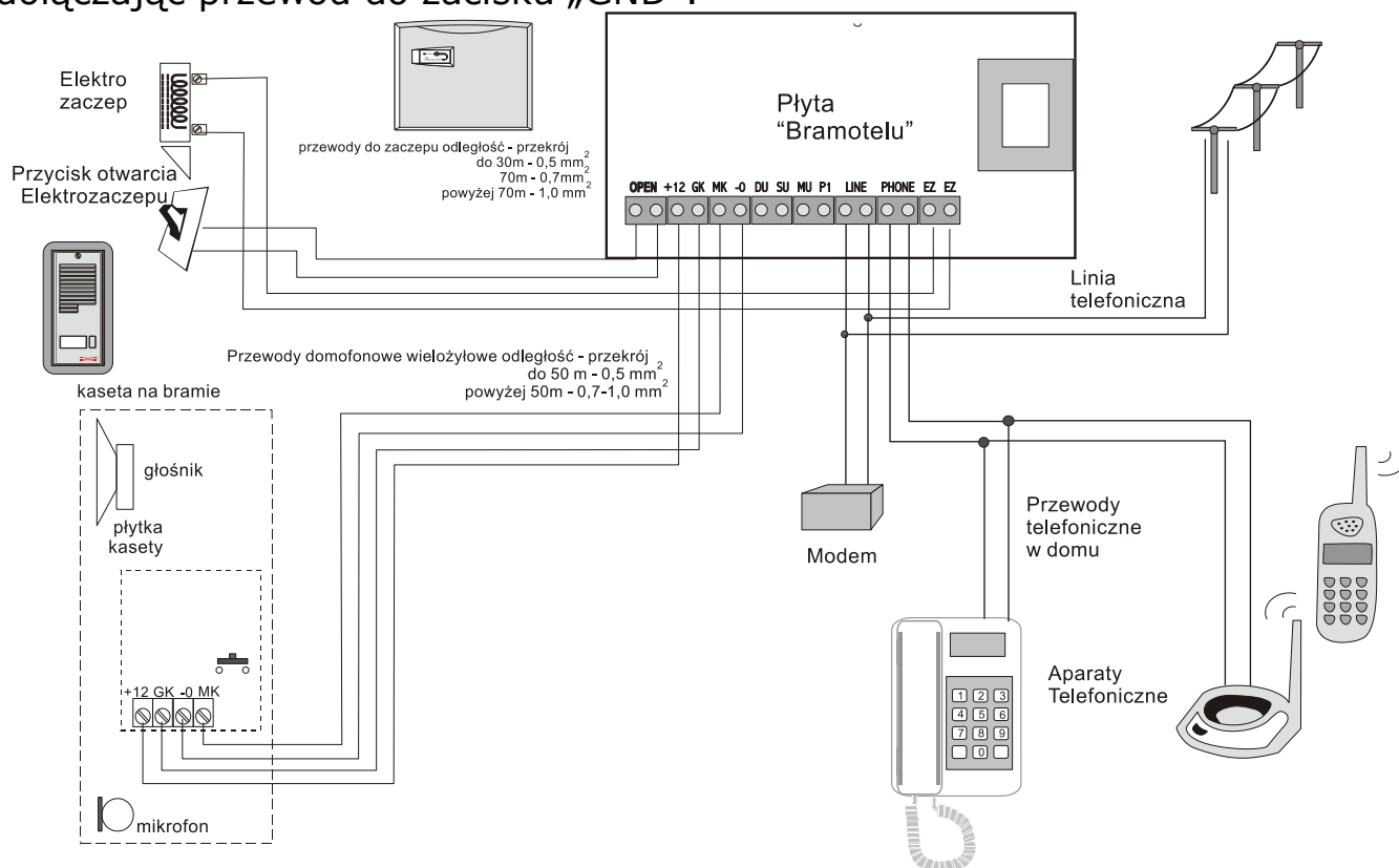
Rys. 2 - Schemat instalacji domofonowej w domku jednorodzinnym.
